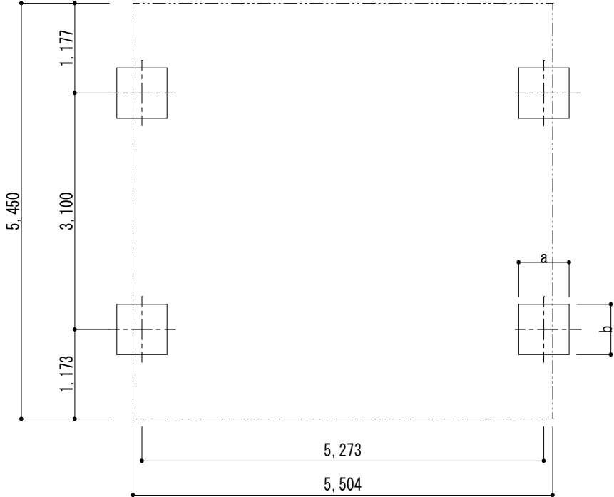
■ 基礎配置図
